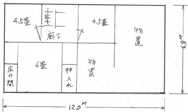
2階間取図
